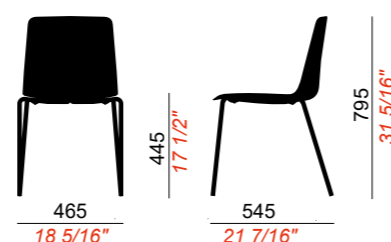
STRUTTURA 4 GAMBE 4 legs frame
