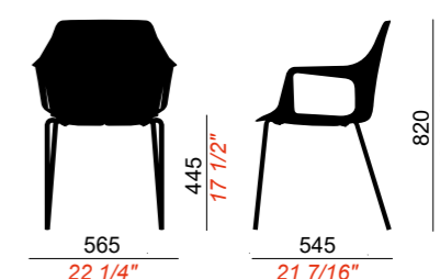
STRUTTURA 4 GAMBE 4 legs frame
