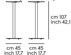
Composit/3 H.107 Base Ø 45 - Col. Ø 8
