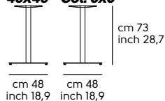
Smart/1 H. 73 Base 48x48 - Col. 6x6
