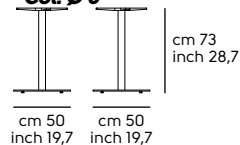
Smart/2 H. 73 Base Ø 50 - Col. Ø 6
