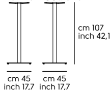
Composit/1 H.107 Base 45x45 - Col. 8x8
