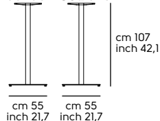
Composit/1 H.107 Base 55x55 - Col. 8x8
