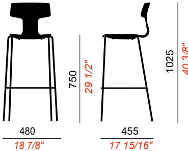
STRUTTURA 4 GAMBE H:750 4 LEGS FRAME H:750
