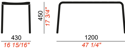
STRUTTURA 4 GAMBE 4 LEGS FRAME
